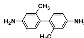
m-TB(Cas No.84-67-3, mp 103°C)
