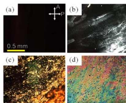
Fig. 2 Polarized optical microscope images of (a) 40 wt% BPDO, (b) 50 wt% BPDO, (c) 40 wt% BPDE, (d) 50 wt% BPDE in NMP.
